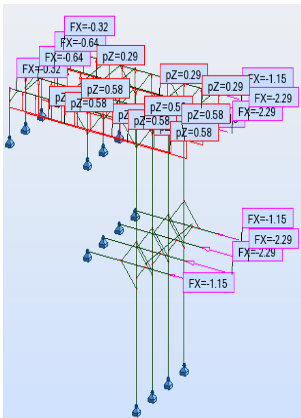
WIATR1 ( \gamma=1,50 )
