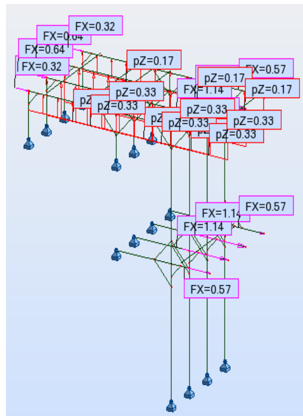
WIATR2 ( \gamma=1,50 )
